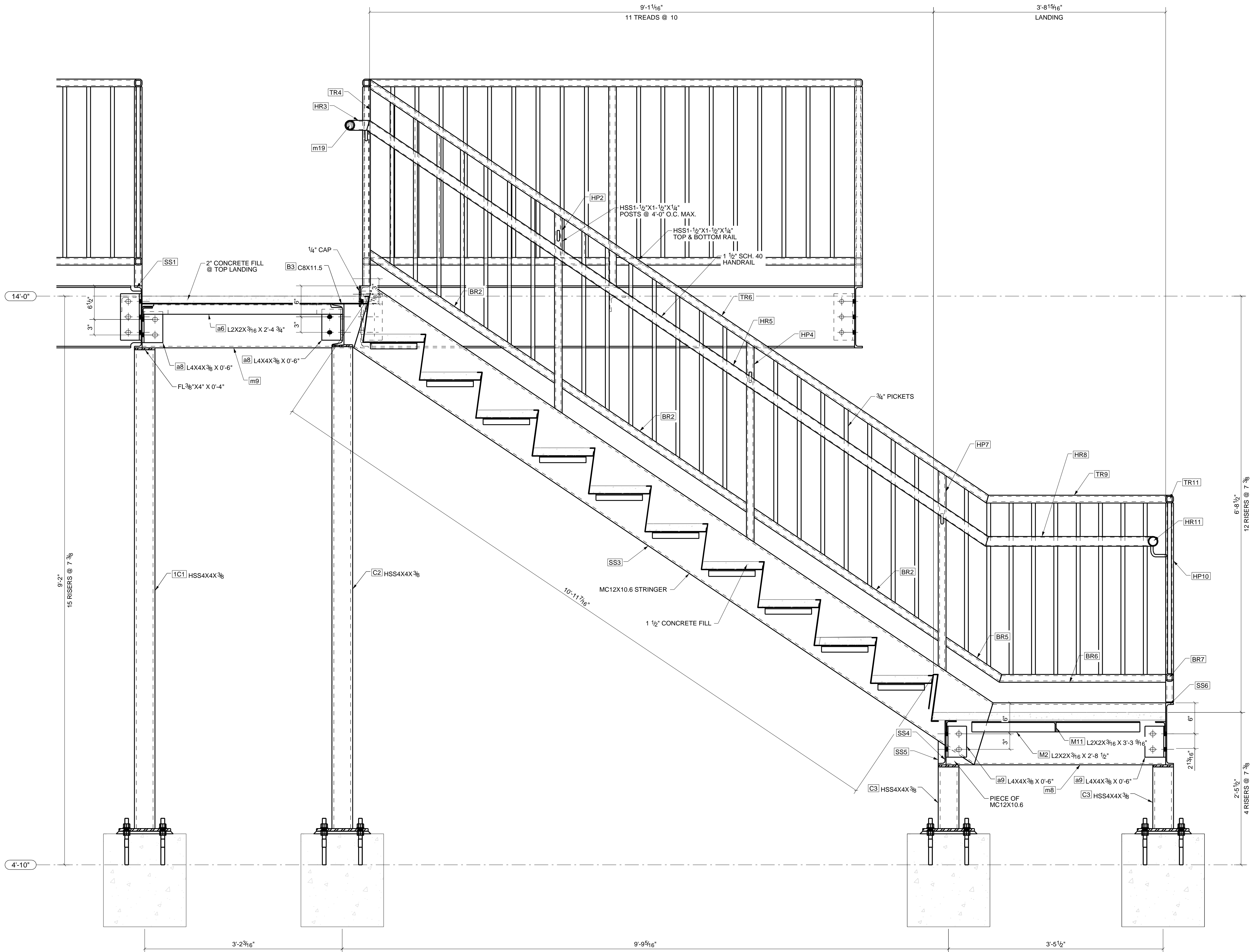
3-3 SCALE: 1/8" = 1'-0"
